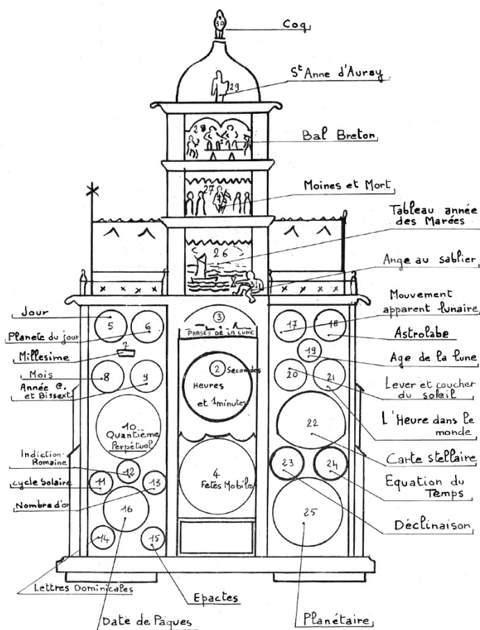
Figure 1. Indications de l'horloge de Vachey.
